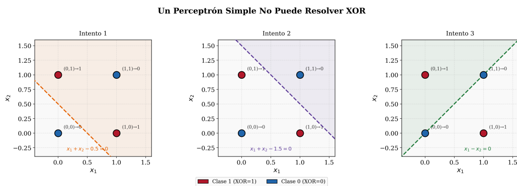
Figura 7.6: Múltiples intentos fallidos para encontrar un hiperplano que permita separar las clases del problema XOR.
