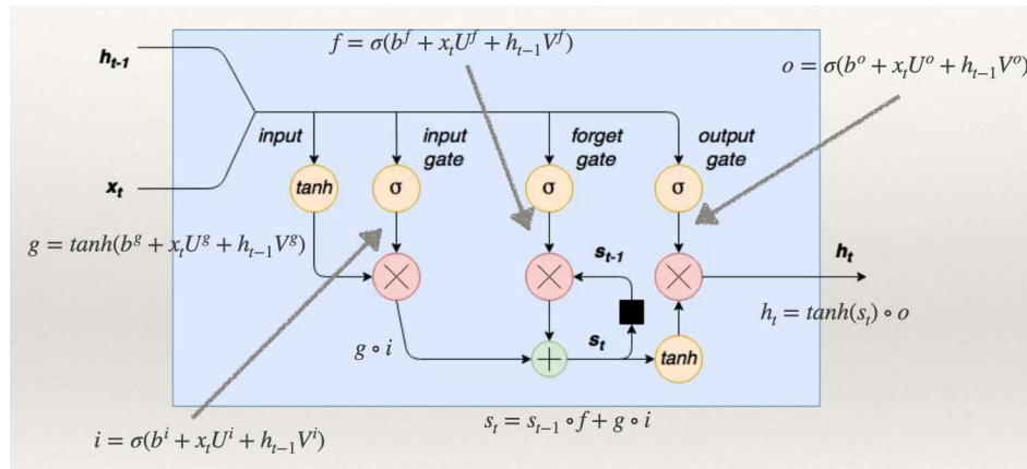
Figura 21.2: Las redes LSTM, Long Short Term Memory, fueron pensadas específicamente para poder superar el problema del vanishing/exploding gradient con un mecanismo de activación de una memoria interna para lograr cadenas de inferencia causales que acepten muchas capas temporales.
