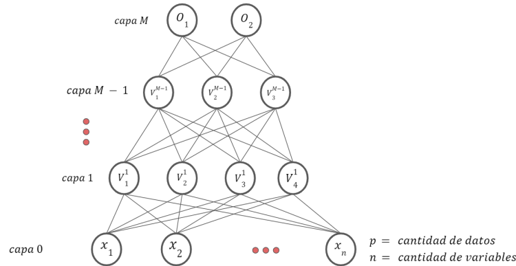
Figura 8.3: Perceptrón multicapa con estructura jerárquica aglomerativa arbitraria. La capa 0 corresponde a la capa de entrada, la capa M corresponde a la capa de salida, y las capas intermedias 1, 2, \dots, m-1 corresponden a las capas ocultas. La letra M indica el número de capas. Cada capa puede tener un número arbitrario de neuronas. Los datos de entrada se representan como un vector x de dimensión n (cantidad de variables o características). El tamaño del conjunto de entrenamiento es p . Para representar las neuronas, se utiliza la letra V para las neuronas de la capa oculta y O para las neuronas de la capa de salida. Para simplificar el esquema, no se incluye el bias, en el cual se hará hincapié más adelante.
