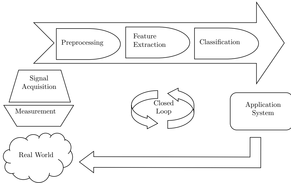
Figura 10.3: Arquitectura General de un Sistema de Aprendizaje Automático
