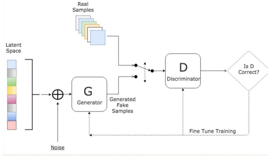
Figura 20.2: Arquitectura de una red GAN, compuesta por una red Generadora y otra Discriminadora que juegan un juego adversarial.
