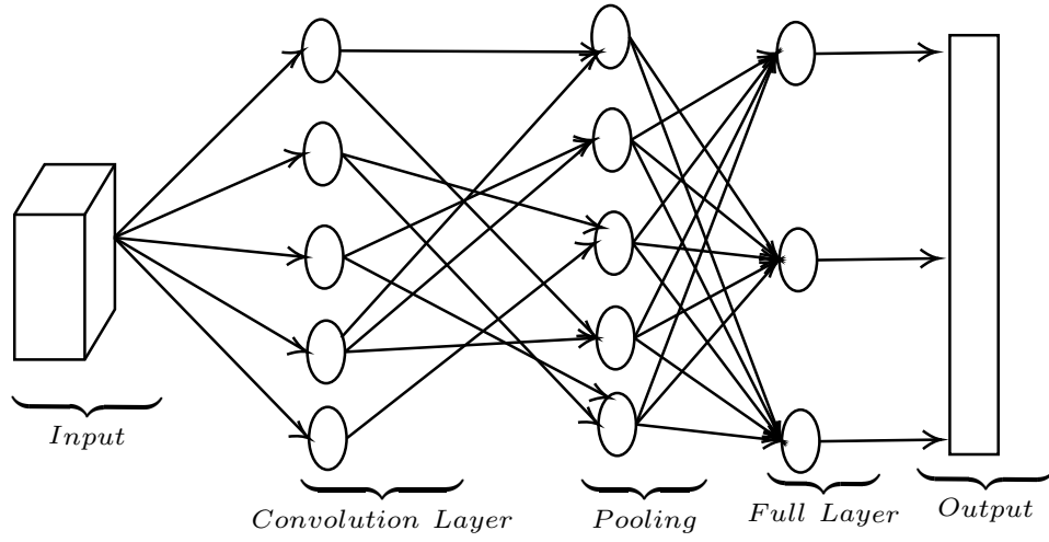
Figura 19.7: Estructura general de una red convolutacional con sus diferentes capas.
