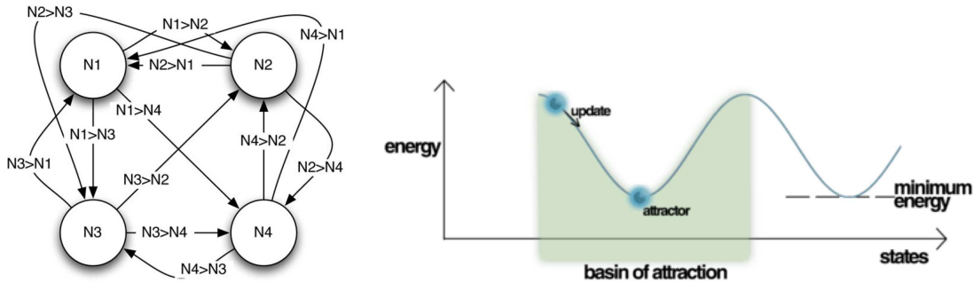
Figura 14.3: Red de Hopfield donde todas las salidas son las entradas de las otras neuronas. El estado de la red puede capturarse con una función de costo/energía que busca minimizarse ante cualquier perturbación (la entrada) y en los valles están los patrones aprendidos.
