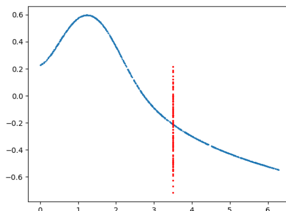
Figura 18.6: Una función seno \sin(\cdot) estocástica. En azul se muestran el promedio de los valores generados por la función. En 3.5 en rojo se muestran todas las instancias particulares generadas para ese punto.
