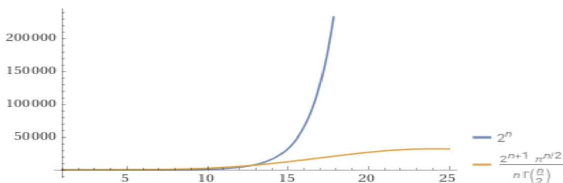
(a) Hiperesfera
