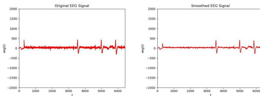
Figura 19.2: A la izquierda una señal de un sensor de electrofisiología que es suavizada con un filtro convolucional del moving average.
