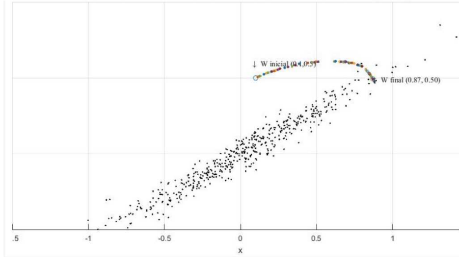
Figura 15.2: Simulación de una neurona lineal con 2 entradas y actualizando w según la regla de Oja. Se ve como el peso se desplaza hacia el eje correspondiente a la mayor variabilidad de los datos.
