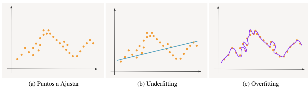
Figura 9.3: Niveles de ajuste sobre un conjunto de puntos. Underfitting se da cuando la curva de ajuste no capture bien el patrón inherente en los puntos (en este caso una curva). Por el contrario, cuando el ajuste es milimétrico, la curva captura el ruido natural en los datos y pierde fuerza de generalización.
