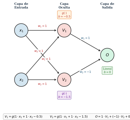
Figura 8.2: Arquitectura de un Perceptrón multicapa para resolver el problema XOR. El esquema corresponde a la red cuya arquitectura da el comportamiento mostrado en la figura 8.1. La función de activación utilizada es la función escalón, denotada por \theta .
