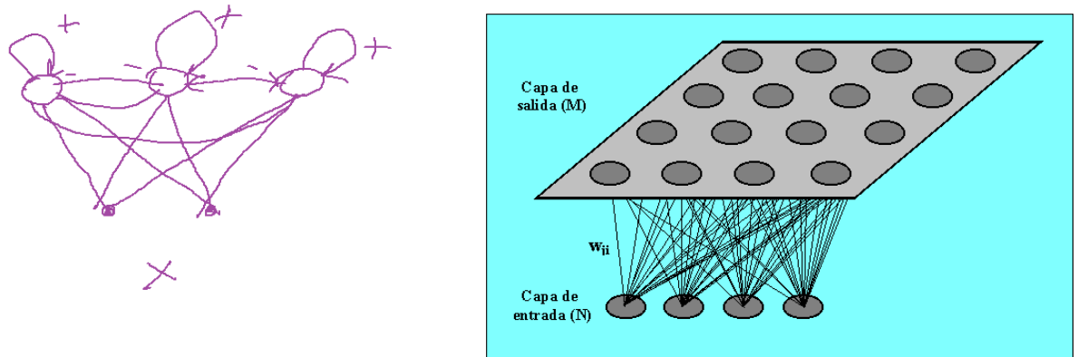
Figura 13.2: Mapa autoorganizado, estructura de conexiones de la red y grilla de salida.
