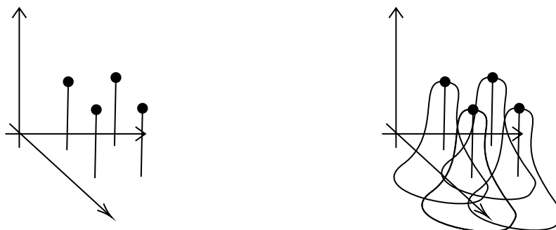
Figura 18.5: En el autoencoder generativo (izq.) cada valor de X tiene una única representación en el espacio latente. En cambio en el autoencoder variacional, se samplean sucesivamente valores alrededor de cada uno de los puntos combinándolos entre ellos, lo que permite que cualquier punto Z tenga alguna representación posible de los valores de X .
