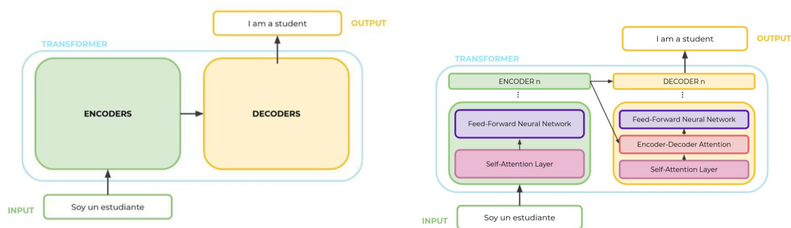
Figura 21.3: Diagrama de componentes básico de un Transformer.
