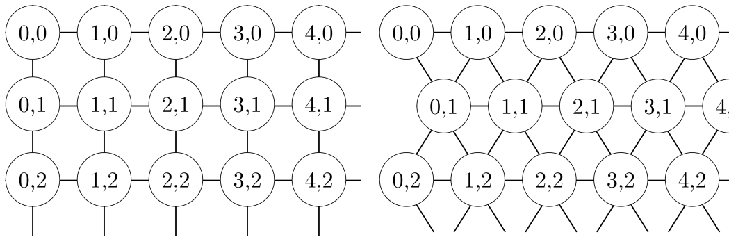
Figura 13.3: Estructuras posibles para la grilla de la red.
