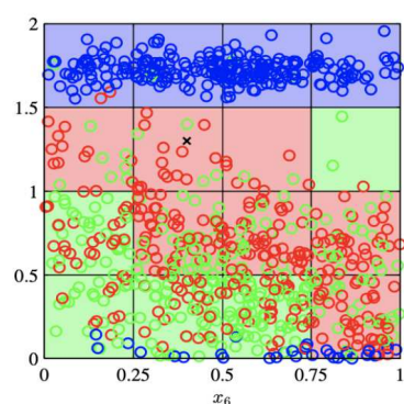
(b) K-NN en 2D
