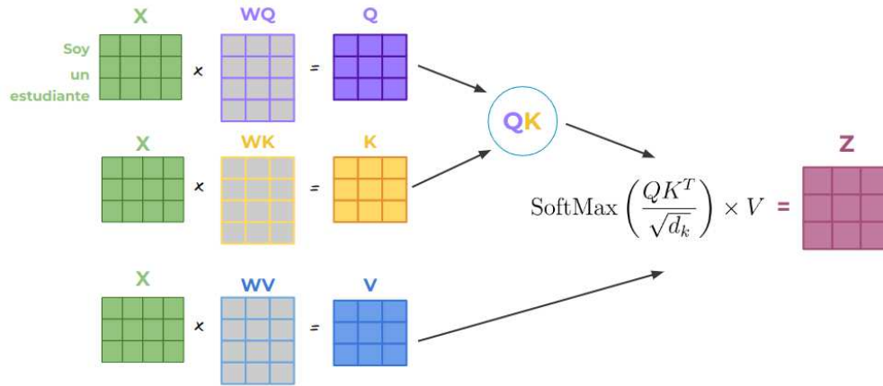
Figura 21.5: Mecanismo básico de Attention y sus componentes.
