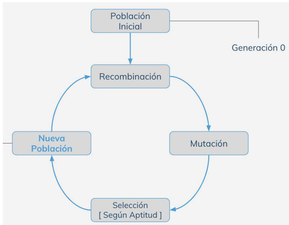
Figura 5.2: Esquema de bloques del patrón básico de un algoritmo genético
