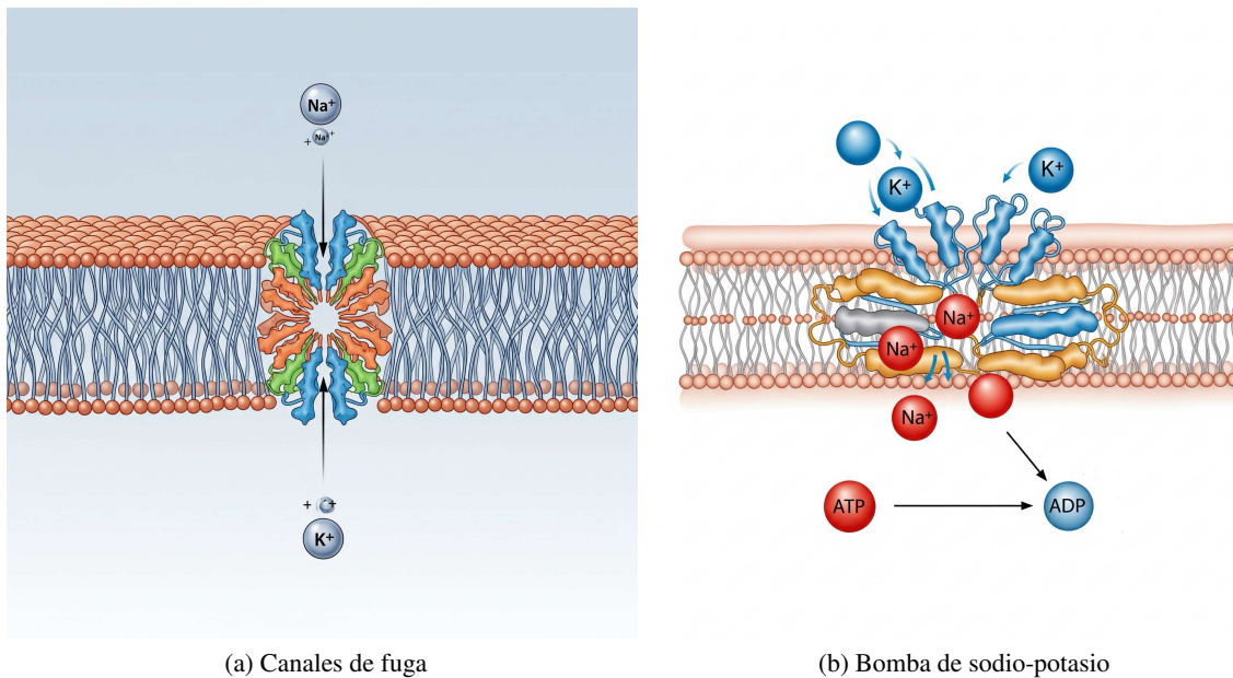
Figura 16.6: Proteínas de membrana que mantienen pasiva y activamente el potencial de membrana.
