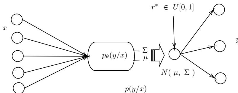
Figura 18.7: Una función \sin(\cdot) estocástica
