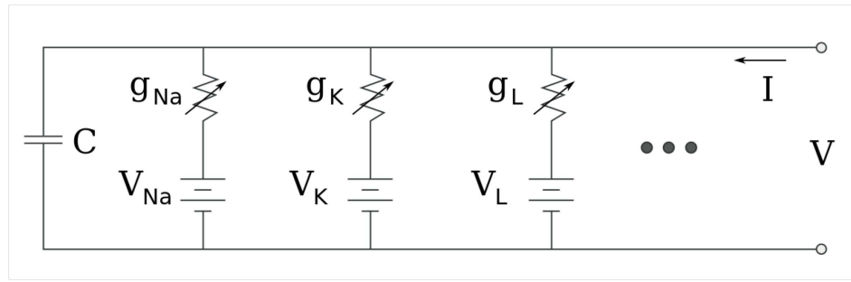
Figura 16.5: Diagrama de Kirchhoff que representa el modelo de Hodgkin-Huxley.
