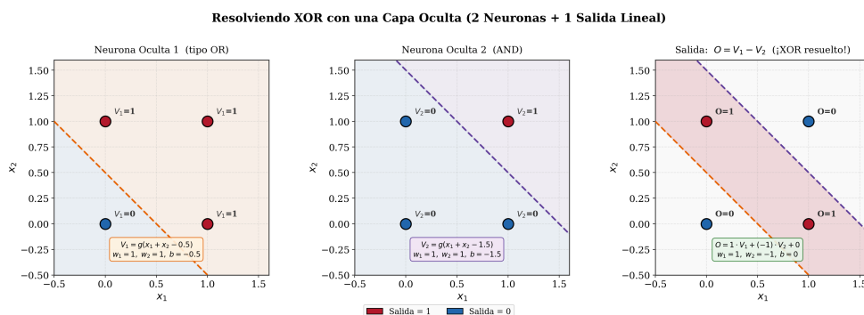
Figura 8.1: Solución al problema XOR utilizando un Perceptrón multicapa. A la izquierda se muestra el hiperplano de separación para la neurona oculta V_1 , y en la imagen central se muestra el hiperplano de separación para la segunda neurona oculta V_2 . A la derecha se muestra el criterio de clasificación de los elementos de entrada, dado por la salida de la neurona O . La función de activación escalón es la que se utiliza en este escenario, denotada por \theta .
